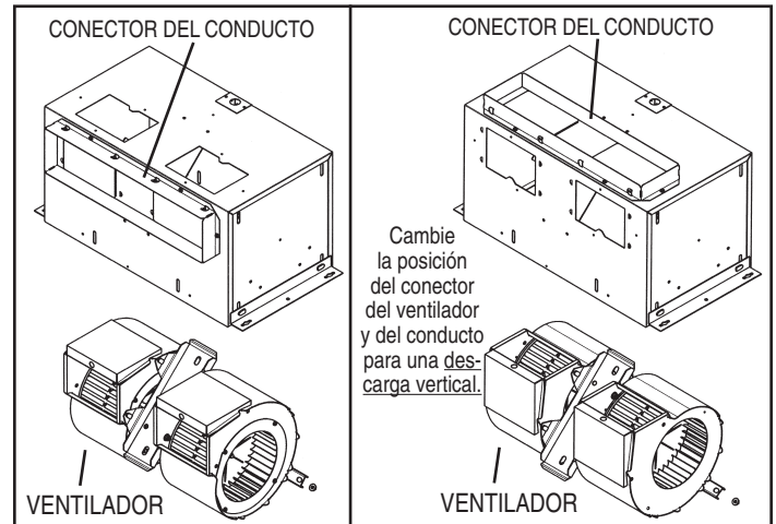
Cambie la posición del conector del ventilador y del conector para una descarga vertical. (enviada de fábrica)
